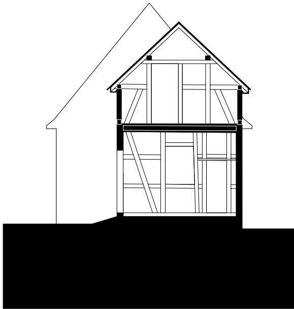
querschnitt a
