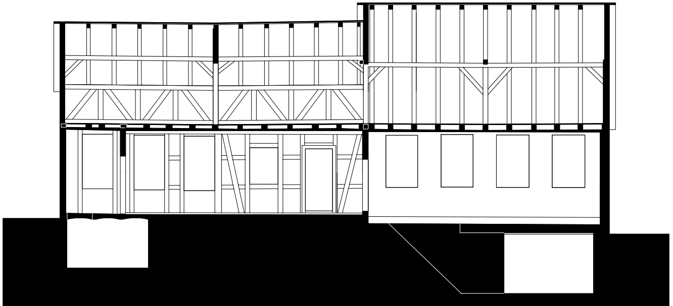
längsschnitt
