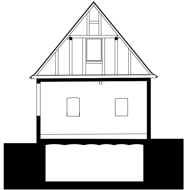
querschnitt b
